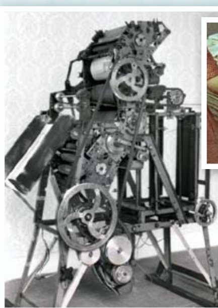
Сконструированная и изготовленная братьями печатная офсетная машина. Производительность — 120 листов в минуту, 400 Евангелий в день.
